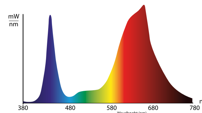
Спектрограмма излучения
