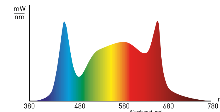
Спектрограмма излучения
