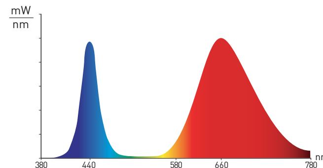
Спектрограмма излучения
